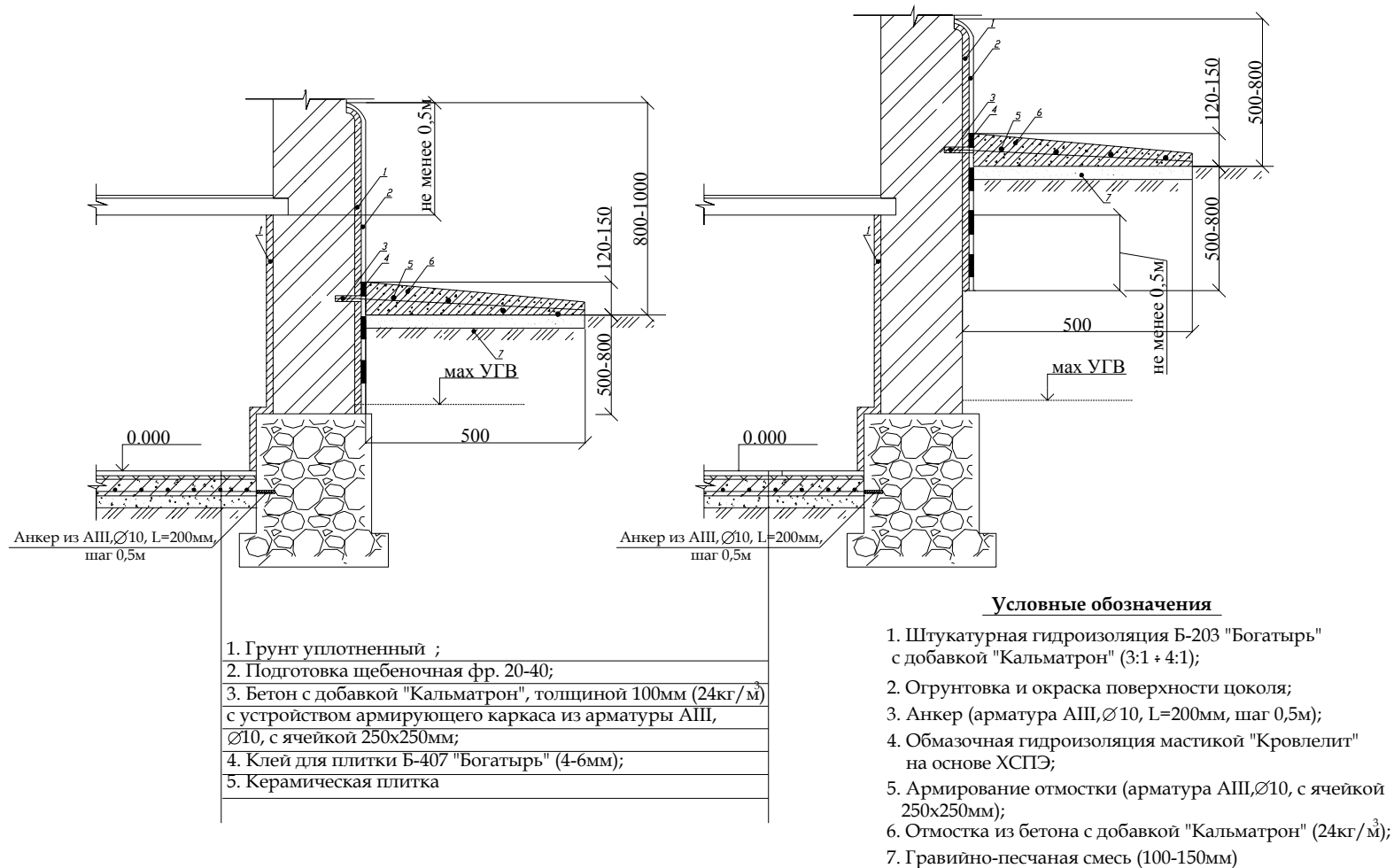
Рис. 3. Конструктивные решения по устройству гидроизоляции с использованием состава проникающего действия «Кальматрон» при реставрации памятников архитектуры
