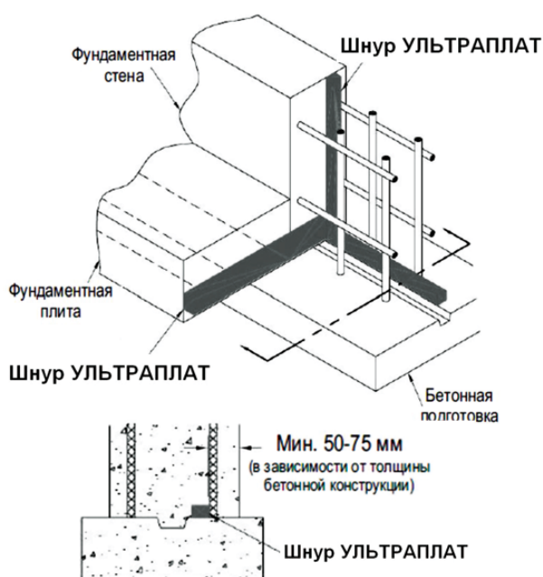
Установка шнура УЛЬТРАПЛАТ на сопрягаемых фундаментных конструкциях
